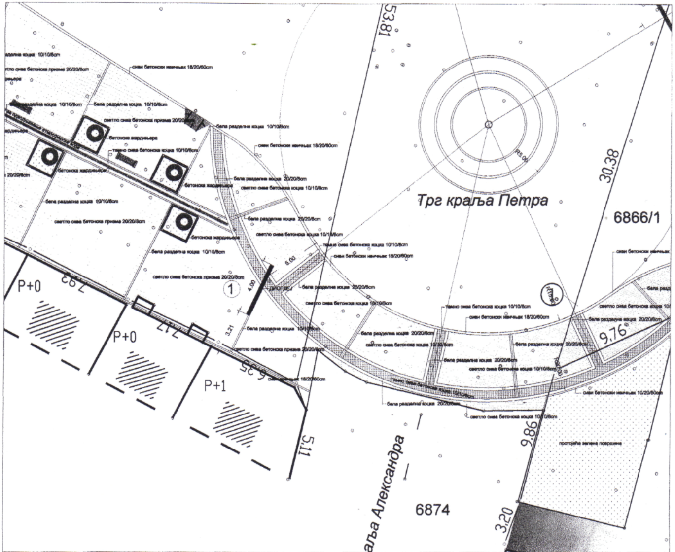
СИТУАЦИЈА P=1:250
